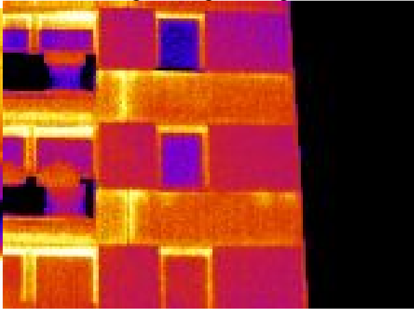
Primer loseg dihtunga kod zgrada
