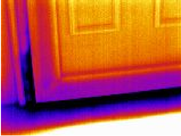
Primer loseg dihtunga na vratima
